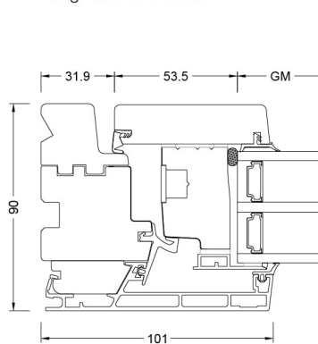
Waagrecht / Horizontal
