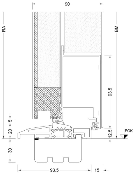
Schnitt unten / Section - bottom
