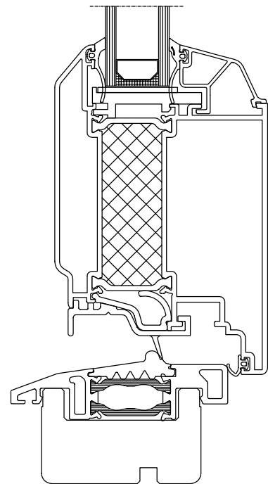
System innenaufgehend
