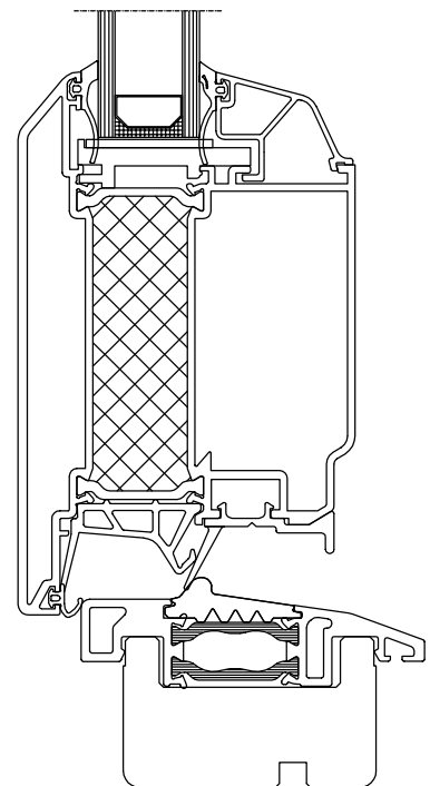
System außenaufgehend
